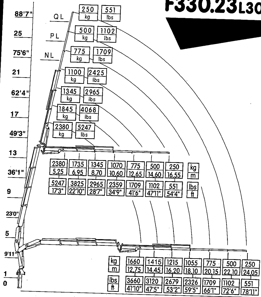
STVLUCHT-TABEL MET LASTBEVEILIGING - DIAGRAM FOR LØFTEMOMENTBRYTER
